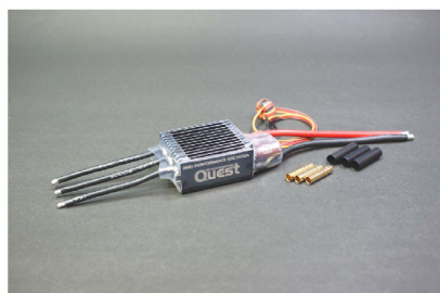
QP0016 ESC-H100A ●9,500 電圧 2~6 LiPo (7.4V~22.2V) 連続最大電流 100A 進角設定 1°/7°/15°/30° PWM 8KHz/16KHz 重量 約120
