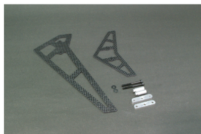
QH0083 カーボン尾翼セット Carbon Tail Fin Set ●4,500
