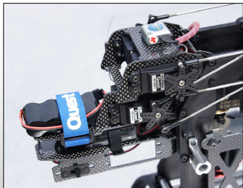
カーボンサーボフレーム
