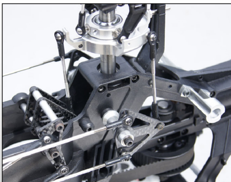
カーボンレバー
